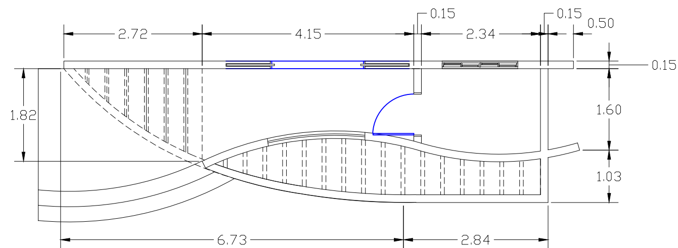
Planta Baixa esc 1/50
