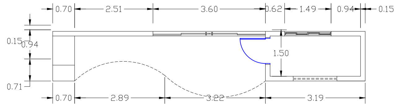
Planta Baixa esc 1/50
